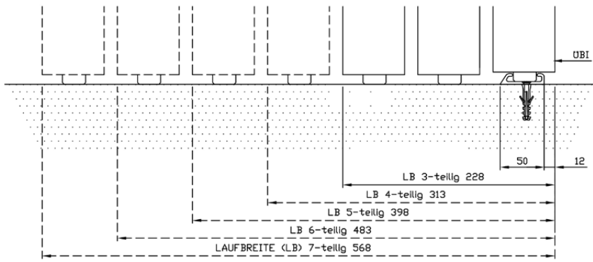
Variante 1: Führungsschiene 50 x 12 mm auf die Terrassenfläche aufgesetzt (einseitig)
