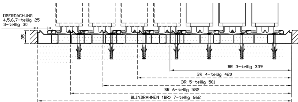
Variante 2: Laufschiene mit Blindrahmen (optional) flächenbündig in die Terrassenfläche versenkt (ein- oder beidseitig)
