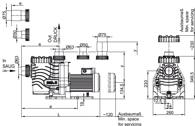
Maßtabelle / Dimension table Maße in mm / Dimensions in mm
